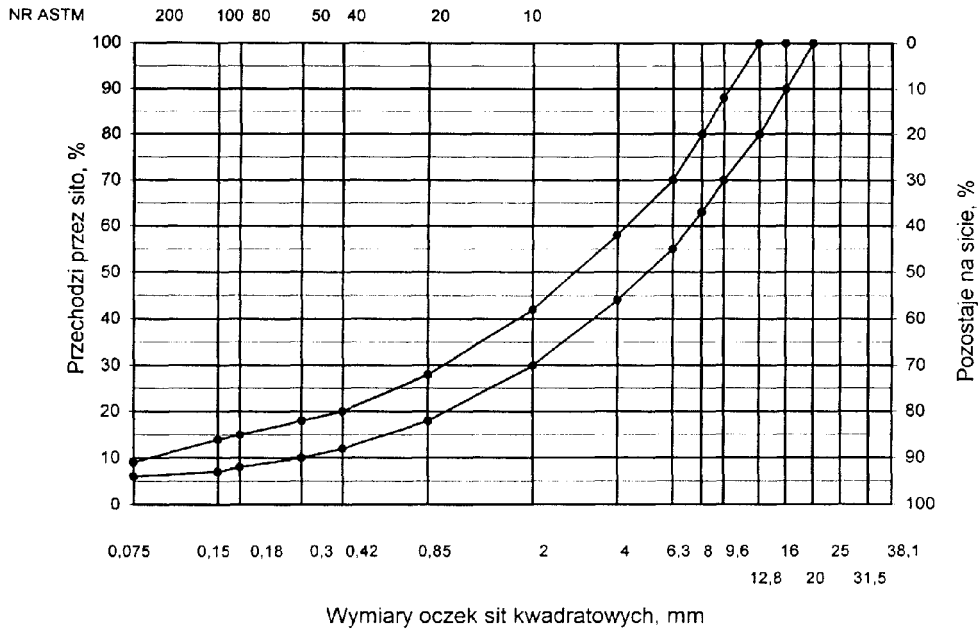
Rys. 6. Krzywe graniczne uziarnienia mieszanki mineralnej BA od 0 do 16 mm do warstwy ściernalnej nawierzchni drogi o obciążeniu
