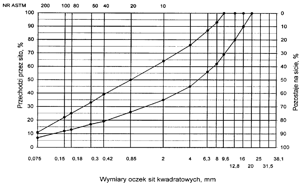
Rys. 2. Krzywe graniczne uziarnienia mieszanki mineralnej BA od 0 do 16mm, od 0 do 12,8 mm do warstwy ściernej nawierzchni drogi o obciążeniu ruchem KR1 lub KR2
