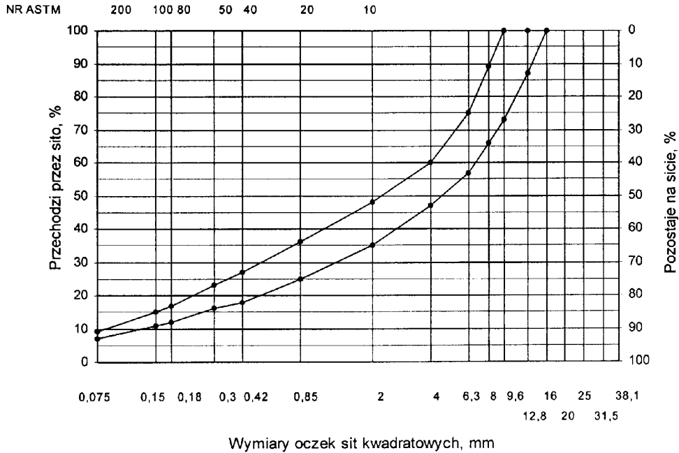
Rys. 6. Krzywe graniczne uziarnienia mieszanki mineralnej BA od 0 do 16 mm do warstwy ściernalnej nawierzchni drogi o obciążeniu
