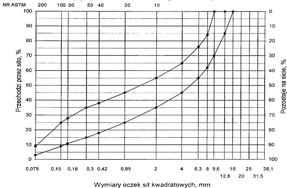
Rys. 9. Krzywe graniczne uziarnienia mieszanki mineralnej BA od 0 do 16 mm do warstwy wiążącej, wyrównawczej i wzmacniającej nawierzchni drogi o obciążeniu ruchem KR1
